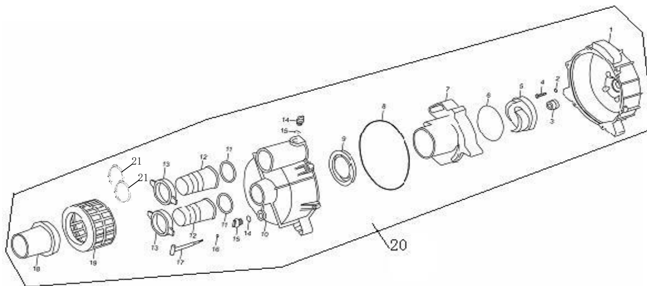
排污泵（TRASH PUMP）
