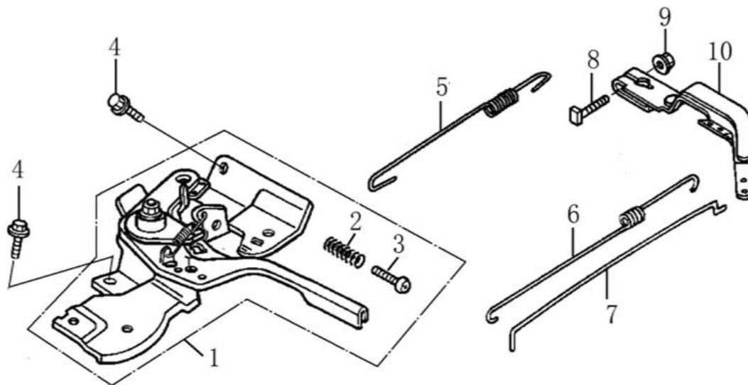
调速控制系统（CONTROL SYSTEM）
