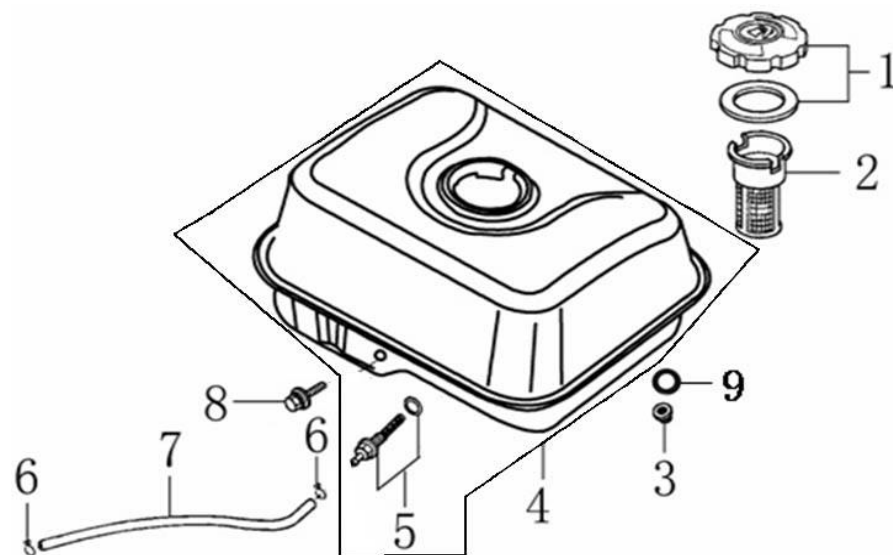
燃油箱 (FUEL TANK)
