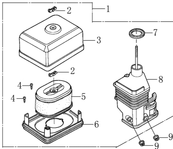
空滤器（AIR CLEANER）
